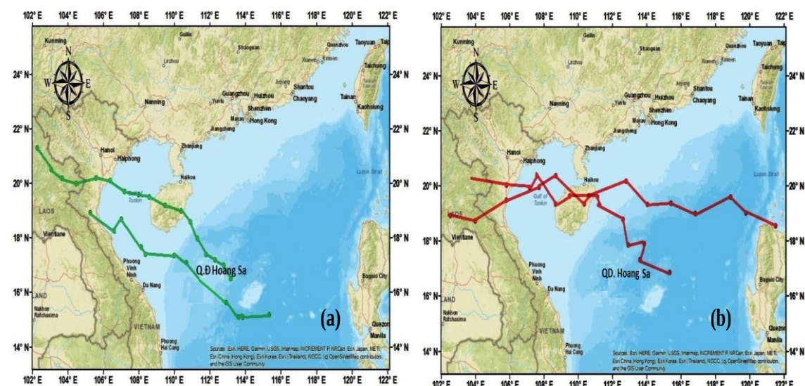
Hình 10. Quỹ đạo 02 cơn bão gây nước dâng lớn nhất tại Hòn Dấu và Hòn Ngự giai đoạn 1951–2010 (a) và 2051–2110 (b). Số liệu bão từ kết quả của mô hình MRI–CGCM3.
