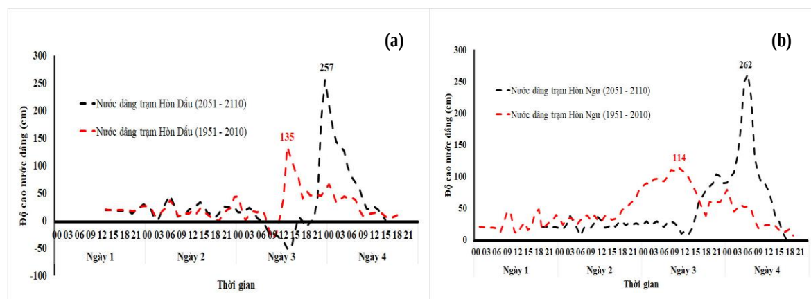
Hình 11. Diễn biến dâng tại trạm Hòn Dấu (a) và Hòn Ngư (b) trong giai đoạn 1951 – 2010 và 2051 – 2110. Số liệu bão từ kết quả của mô hình MRI–CGCM3.
